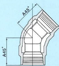
45°エルボ
