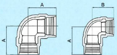
エルボ
